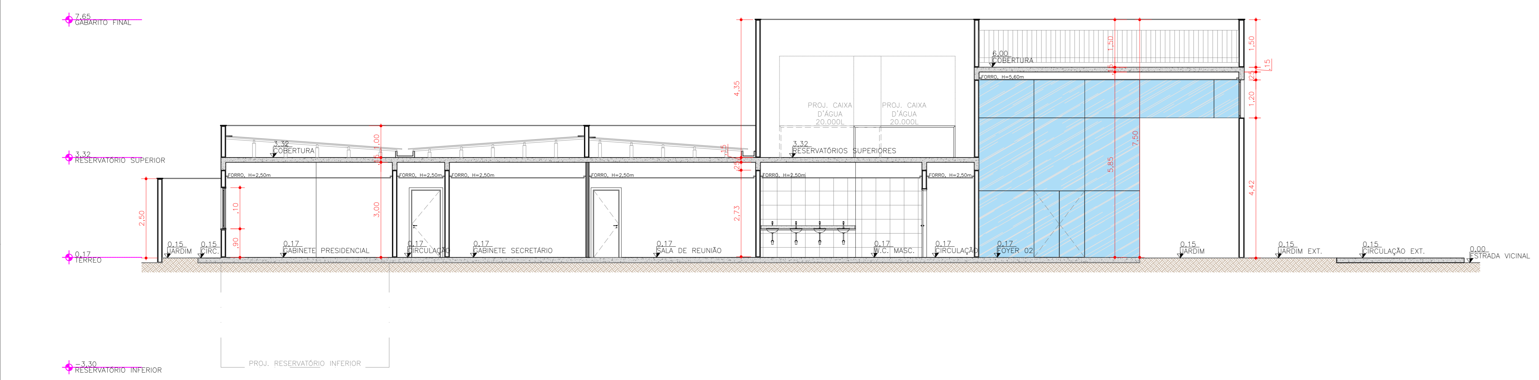
02 CORTE BB ESCALA: 1/75
