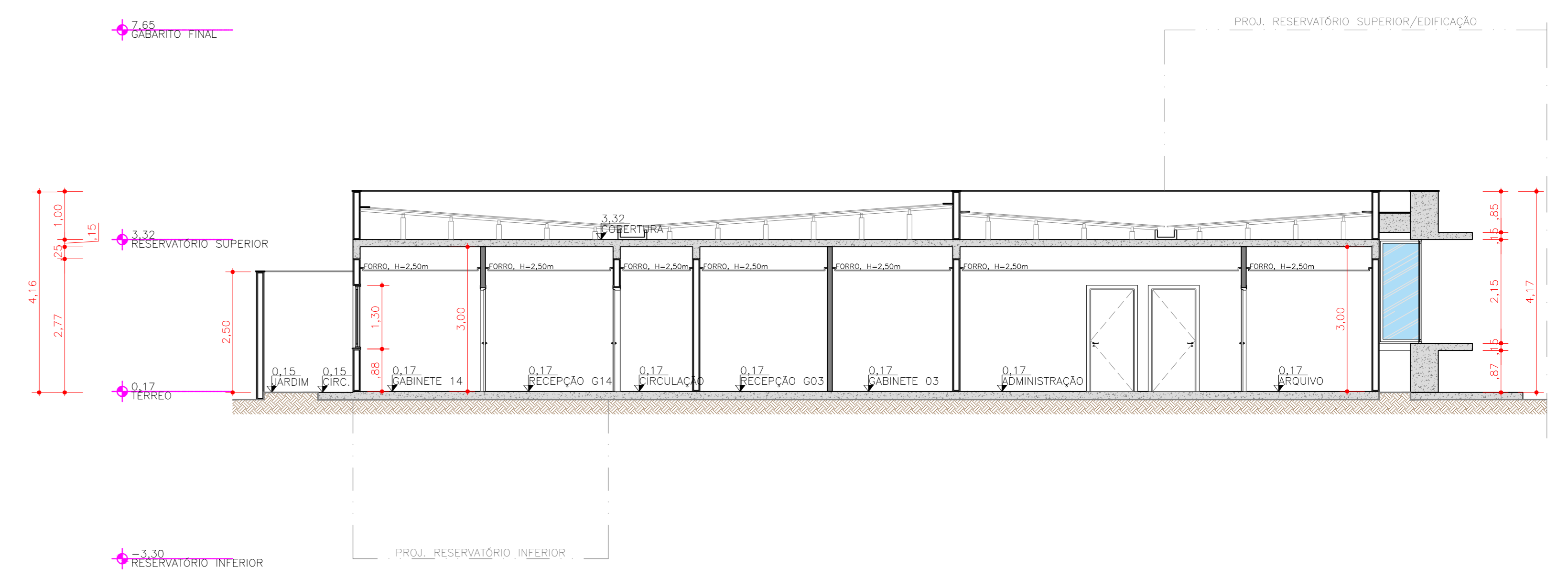
03 CORTE CC ESCALA: 1/75
